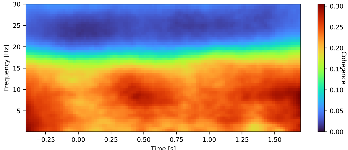
8AD (5) - dPFC (9)
